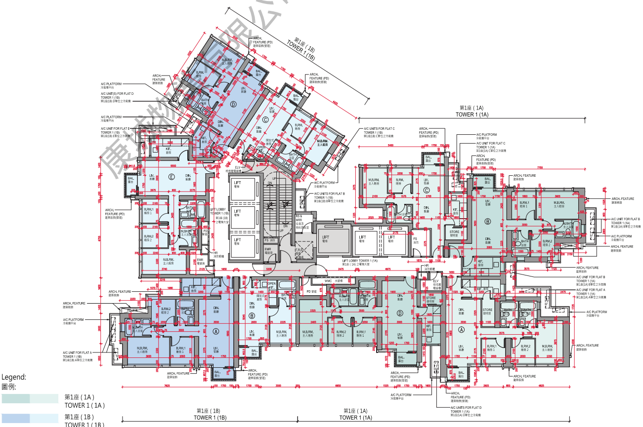
TOWER 1 (1A & 1B) 7/F-12/F AND 15/F-23/F FLOOR PLAN 第1座 (1A & 1B) 7樓至12樓及15樓至23樓樓面平面圖
